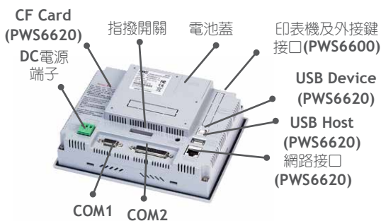
PWS6600/PWS6620背圖
