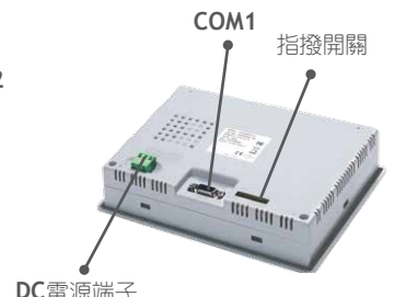
PWS5610背圖
