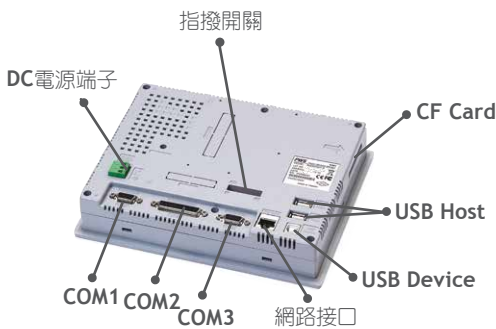
PWS6700/PWS6800背圖
